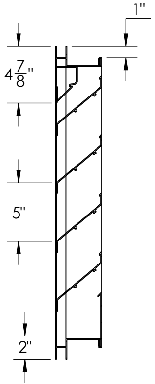
SECTION A-A SCALE 1 : 8
