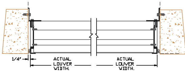
JAMB FRAME
